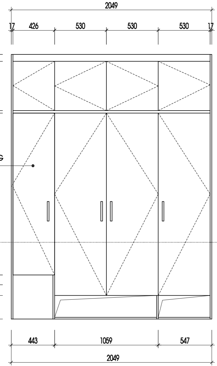
MẶT ĐỨNG
