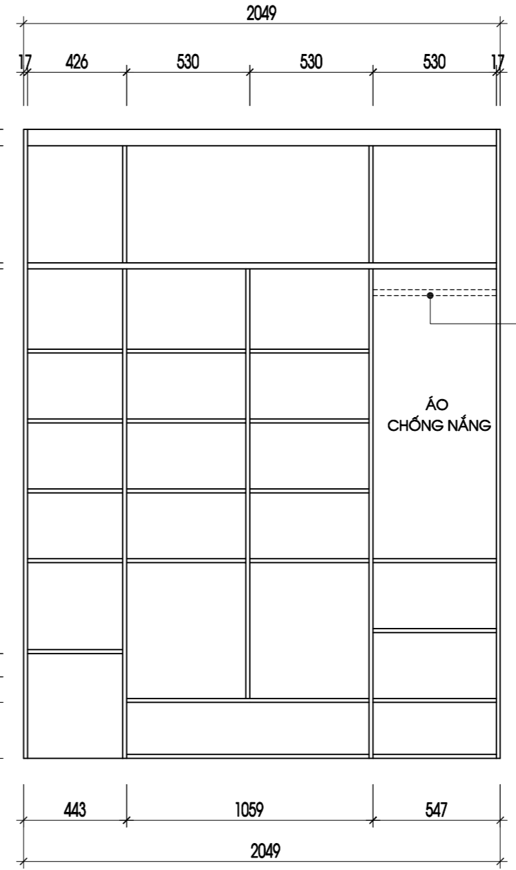
MẶT ĐỨNG BỎ CÁNH
