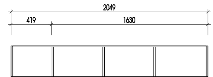
MẶT CẮT 1-1
