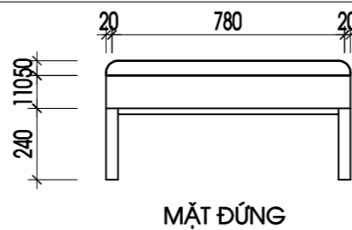
MẶT BÀNG
